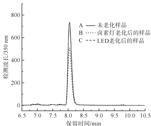
图 3 黄檗在不同光源光老化 360 d 后的高效液相色谱图 Fig. 3 HPLC figure for amur cork after light aging for 360 days under different light sources
