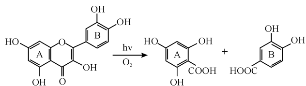
图 5 槲皮素光氧化反应及其可能的产物
