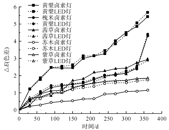
图 2 五种染料在卤素灯及 LED 灯下的常规光老化色差变化曲线
